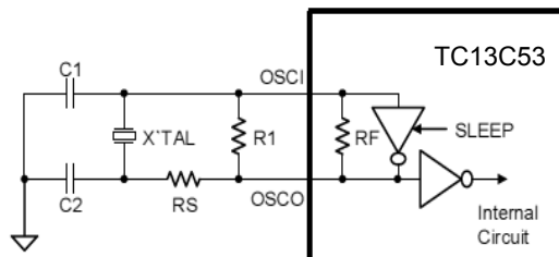
图解 2.6: HF, XT or LF 振荡器模式(晶振操作或陶瓷共鸣器)
