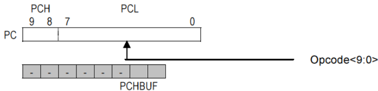
图2.2: 不同的指令调用PC指针跳转方式
