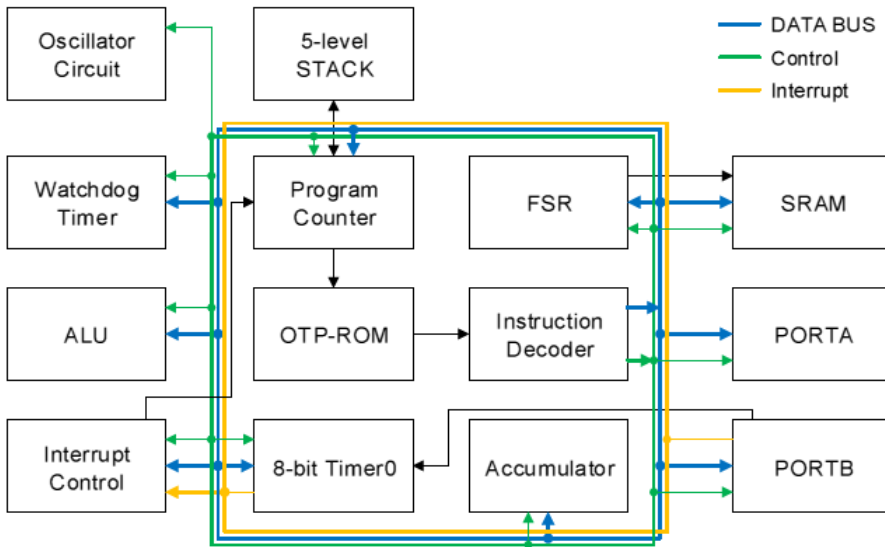
方块图
